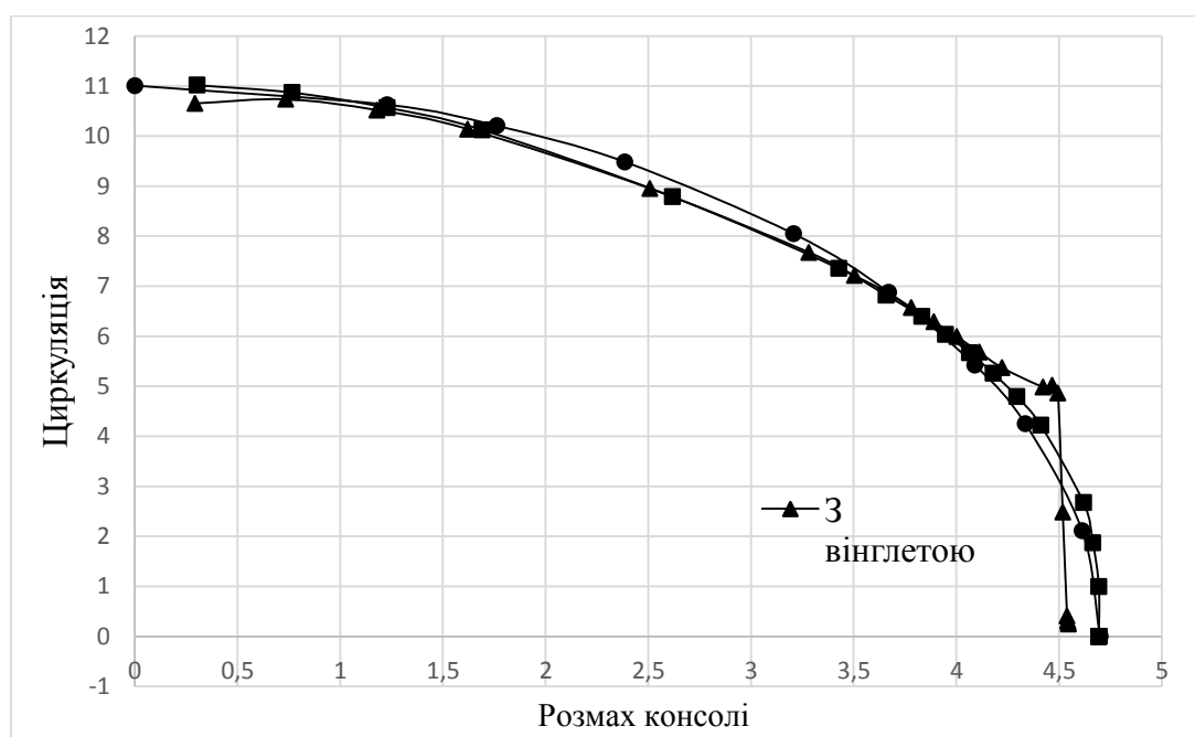
Рис. 3. Розподіл циркуляції по крилу
