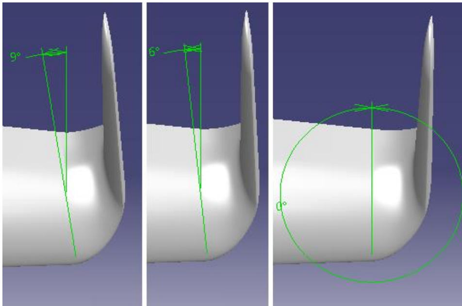
Рис. 2. Кути встановлення адаптивної в'їнглети
